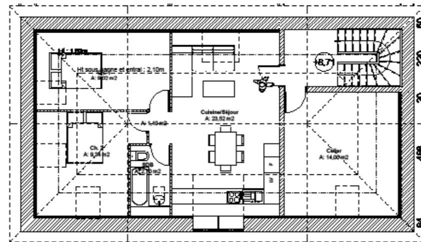
Plan étage courant
